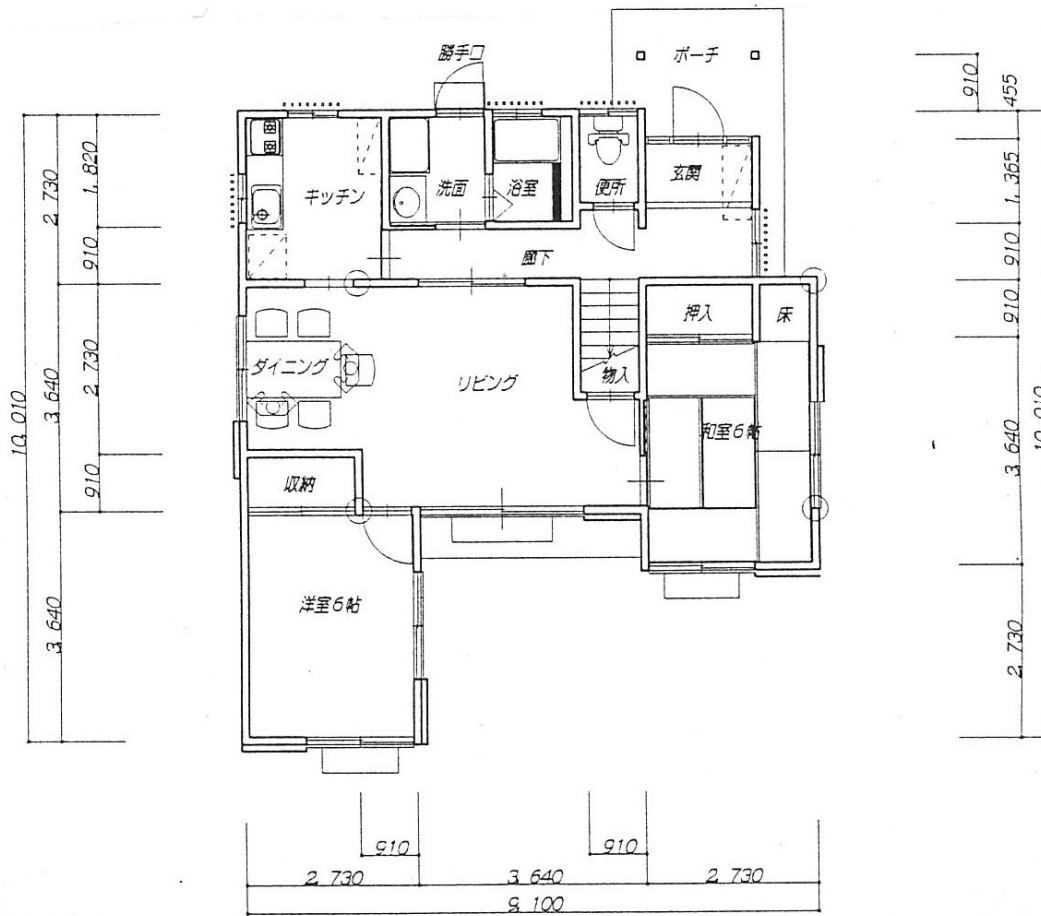
1階平面図
