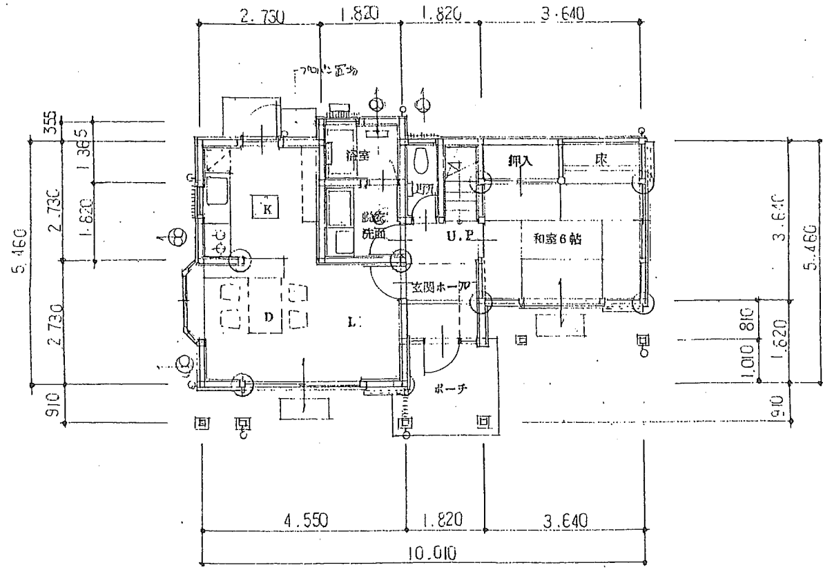
1 階 平 面 図
