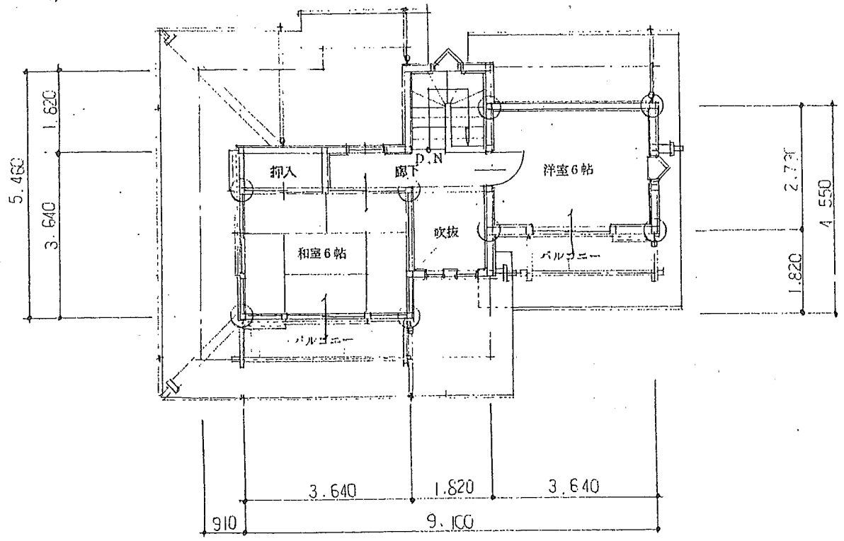
2 階 平 面 図
