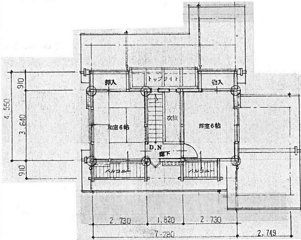
2階平面図
