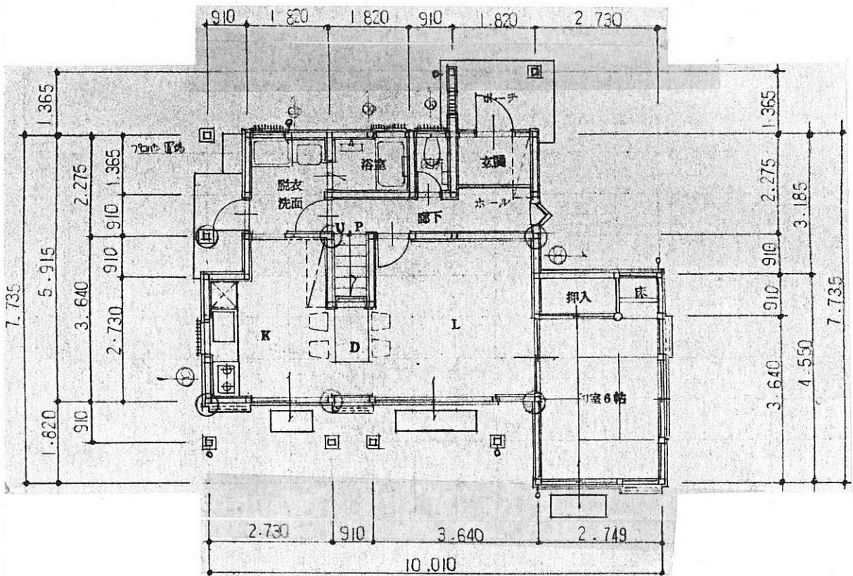
1階平面図
