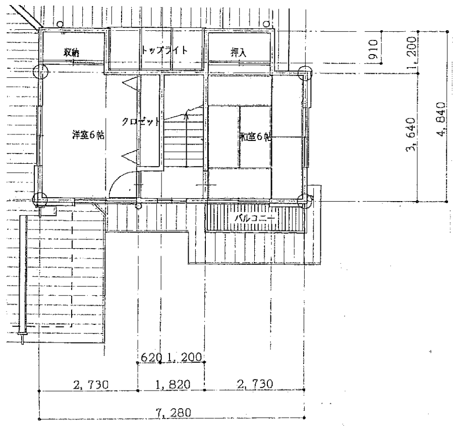
2階平面図
