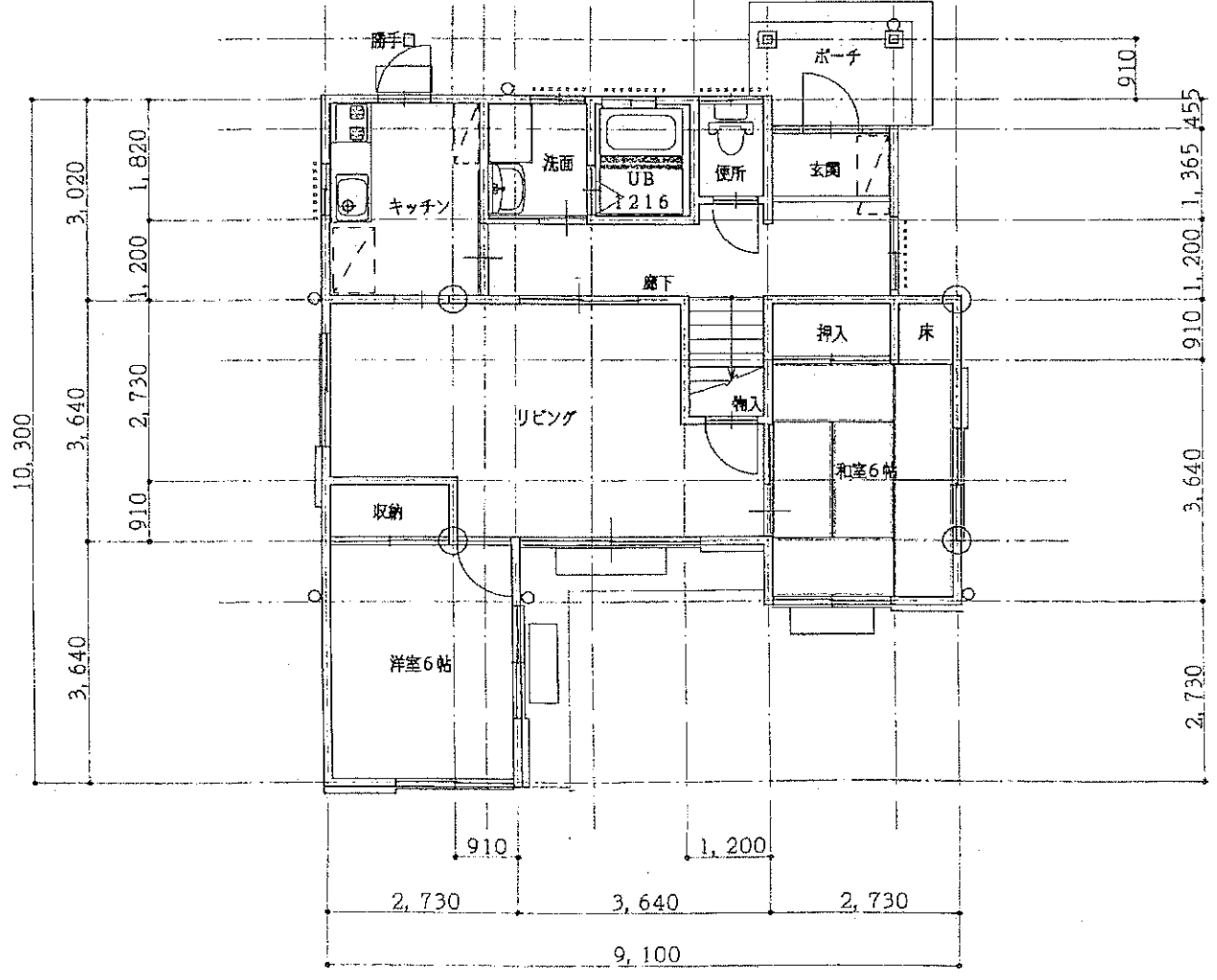
1階平面図
